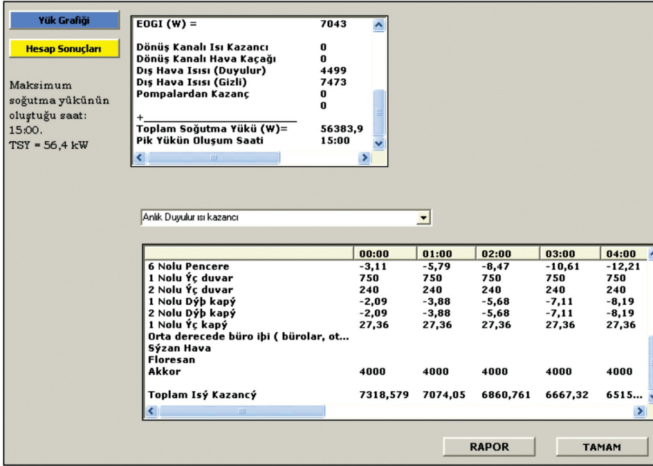
Şekil 13. "Soğutma Yüğü" Sekmesi Altında Açılan Pencere Görüntüsü.
