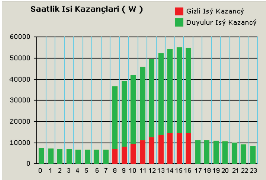
Şekil 14. Soğutma Yüğüne Saatlere Göre Grafik Olarak Gösterilmesi.
