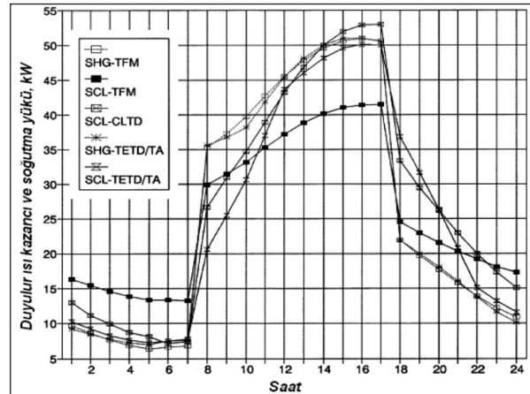
Şekil 1. Duyulur Isı Kazancı ve Soğutma Yüğüünün Hesaplanmasında TFM, CLTD/SCF/CLF ve TETD/TA Yöntemlerinin Karşılaştırılması [5].
